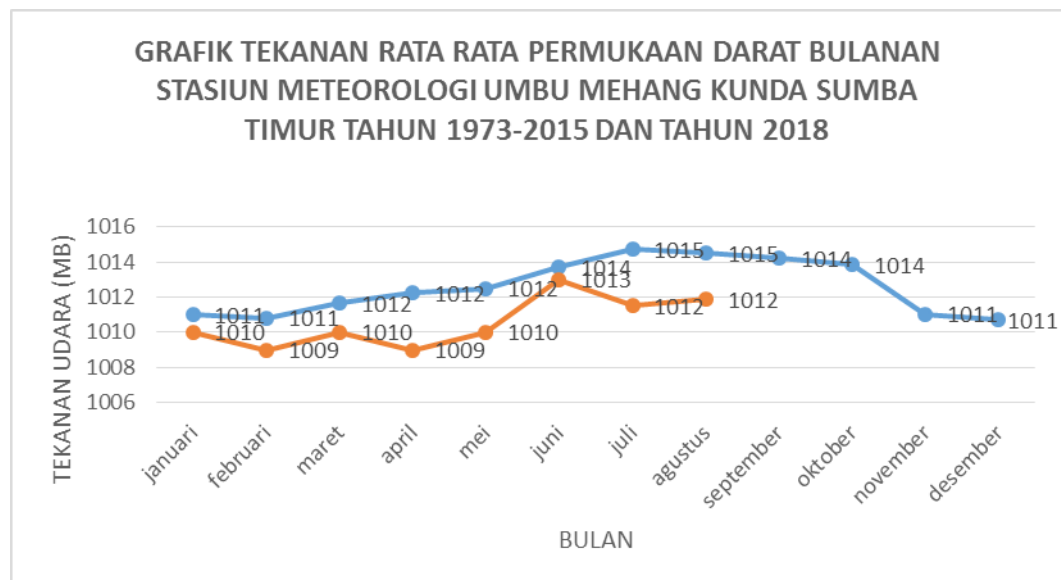
Grafik Tekanan Udara Permukaan Darat
