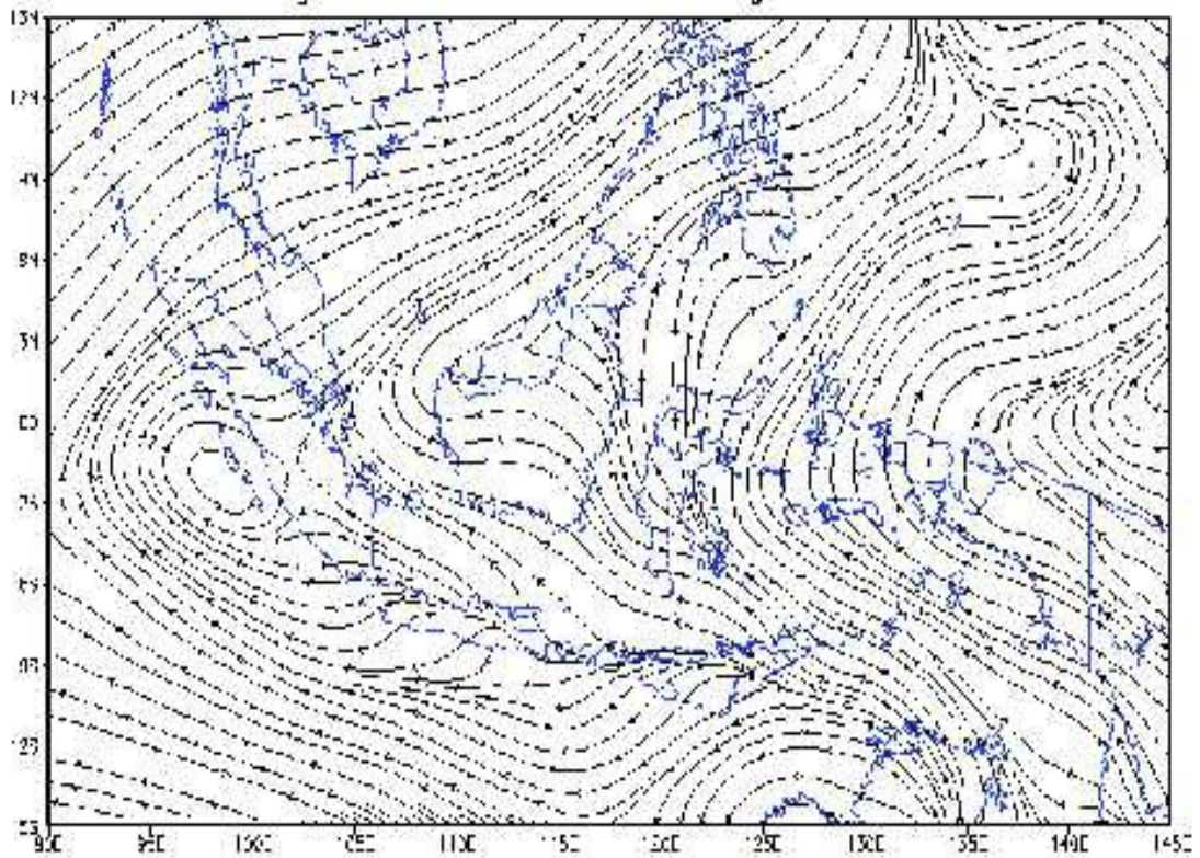
Angin 850mb Dasarian III Agustus 2018
